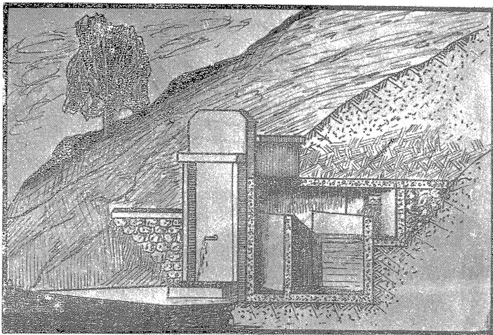
Тип каптаже с чесмом.
